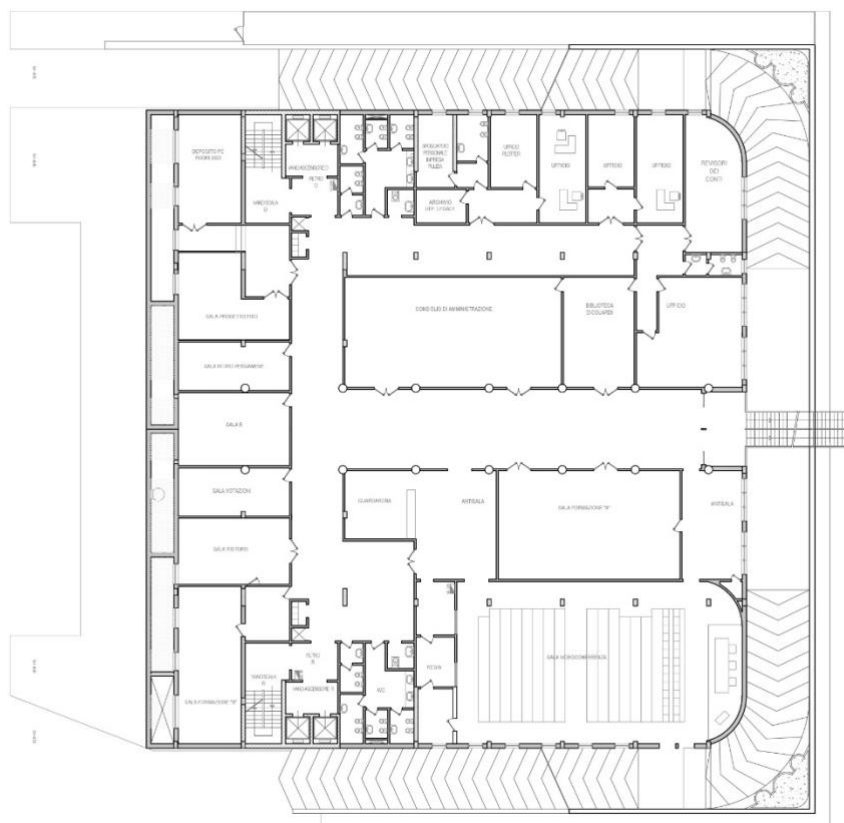
Planimetria Piano -2 (stato dei luoghi)
